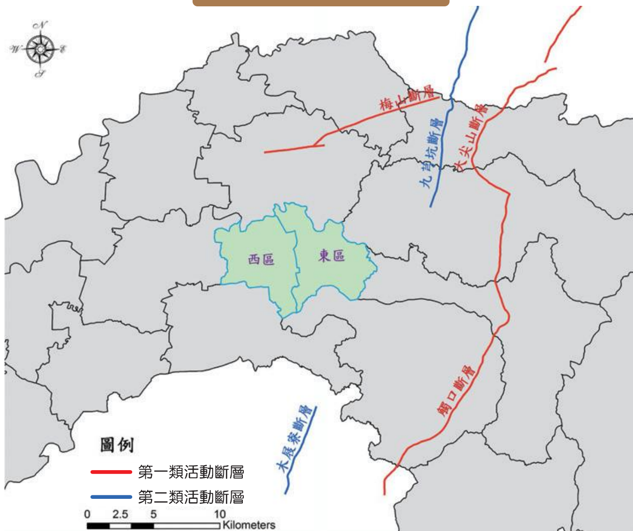
嘉義市鄰近斷層分佈圖
