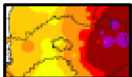
2004年艾利颱風8/23-8/26累積雨量圖
