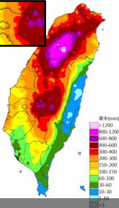
2004年艾利颱風8/23-8/26累積雨量圖
